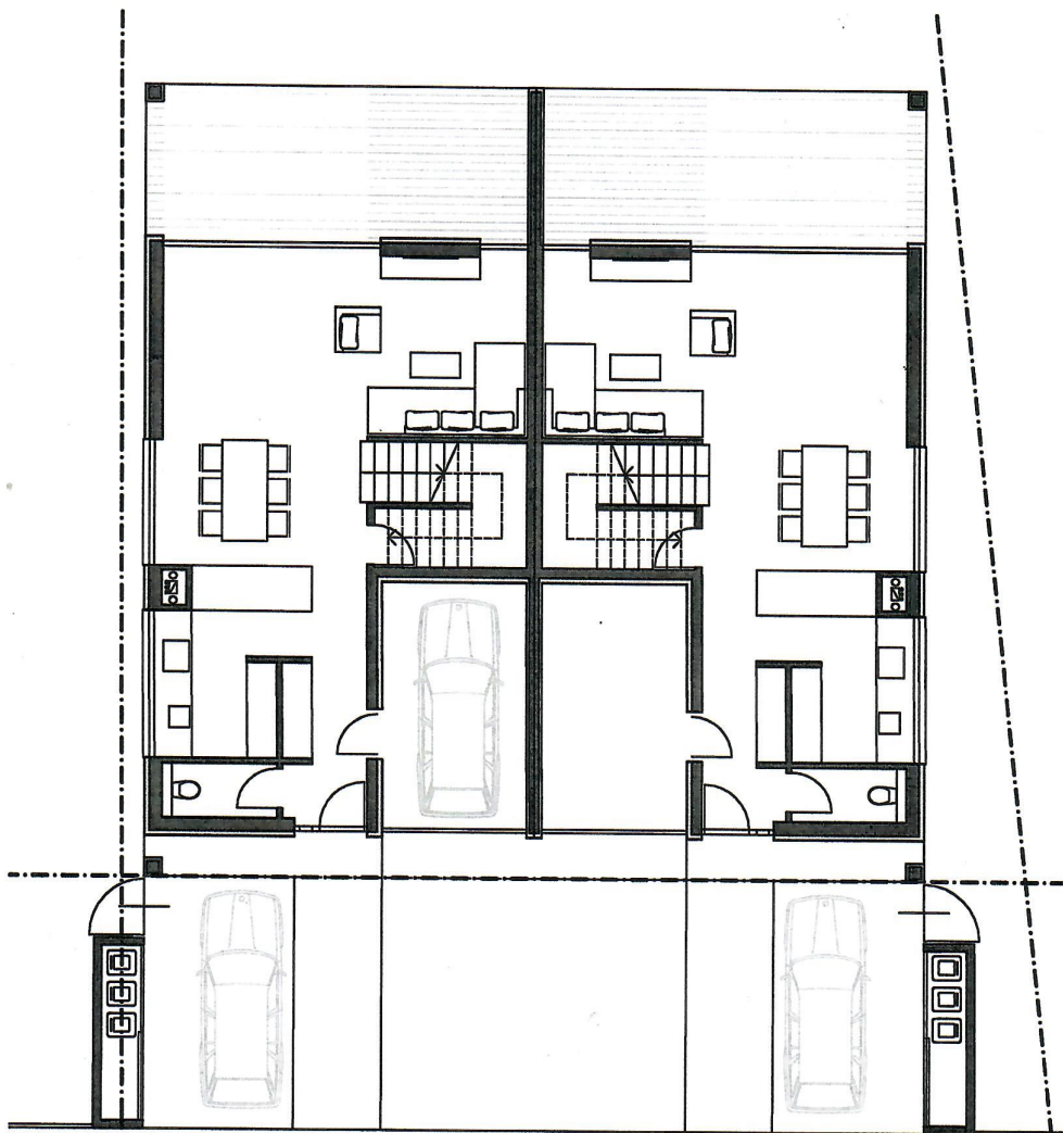
Grundriss Erdgeschoß 1:150
