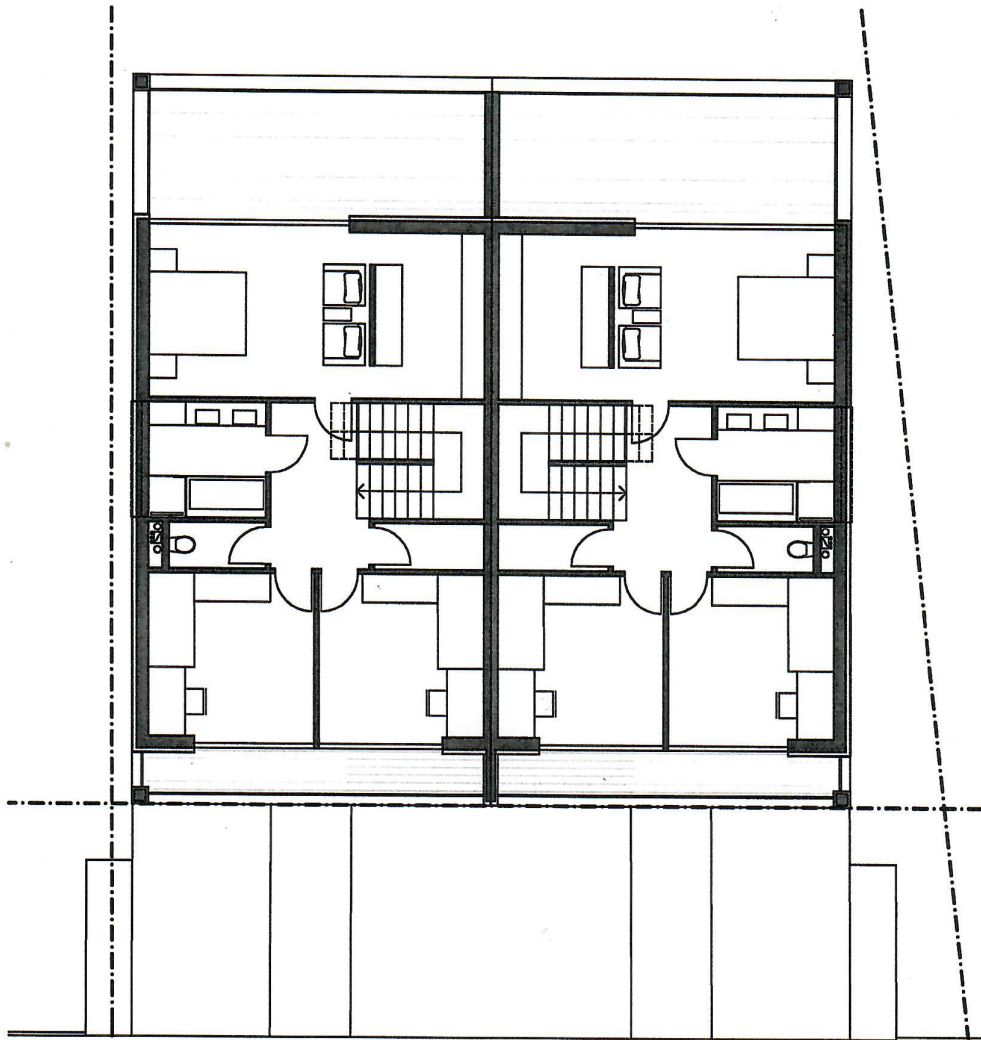
Grundriss Obergeschoß 1:150
